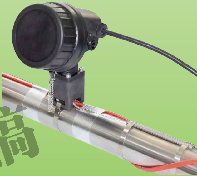
典型的管道安装
